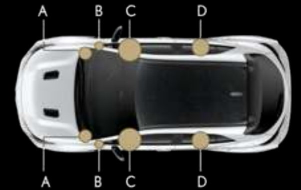
8スピーカーレイアウト A：8cm スコーカー B：2.5cm ツィーター C：17cm ウーハー D：15cm フルレンジ
